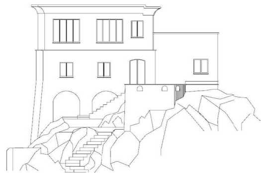
Prospetto est
