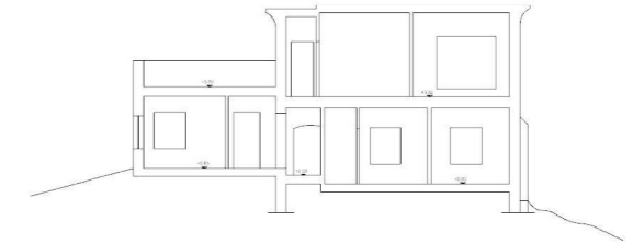
Sezione A-A
